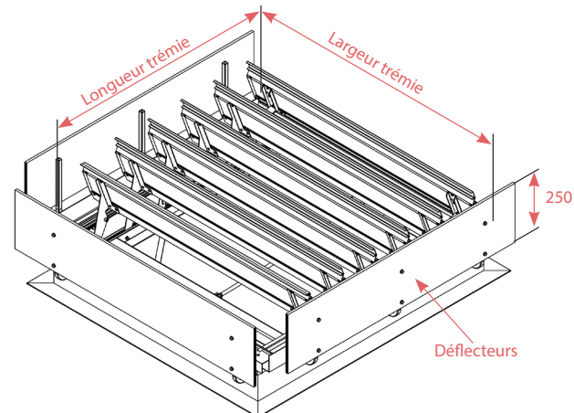
ARCALAM® ÉVOLUÉLEC type Sans Retombée avec déflecteurs
