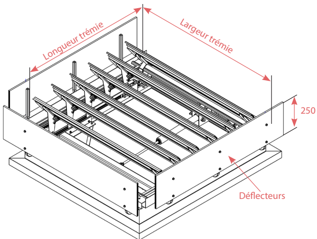
ARCALAM® ÉVOLUÉLEC type Sans Retombée avec déflecteurs
